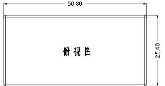
标准型 50.8*25.4*12.7mm
