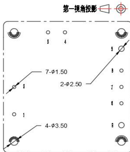
推荐PCB开槽尺寸
