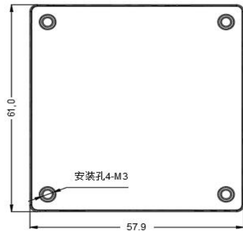
标准型 61.0*57.9*12.7mm
