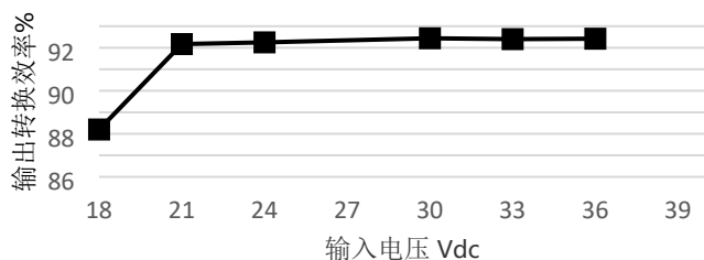
额定输出/降额曲线
