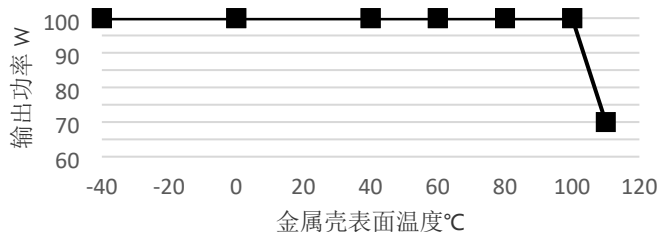
24V 输入降额曲线图
