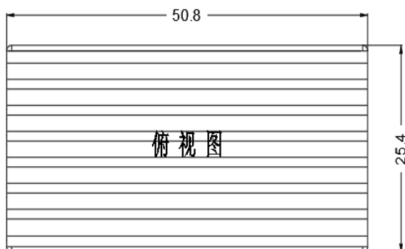
标准型+散热器 50.8*25.4*22.7mm
