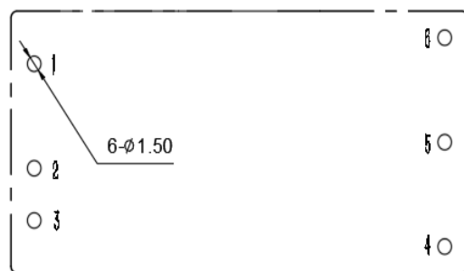
推荐PCB开槽尺寸
