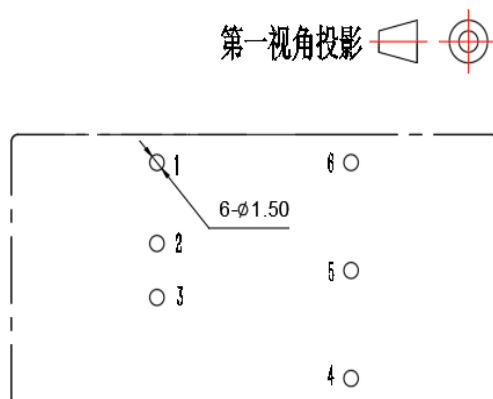
推荐PCB开槽尺寸
