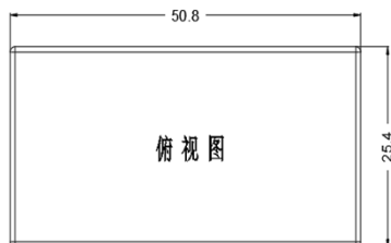
标准型 50.8*25.4*12.7mm
