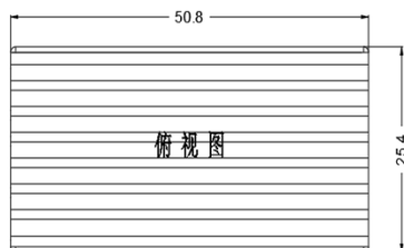
标准型+散热器 50.8*25.4*22.7mm
