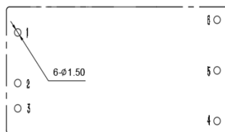
推荐PCB开槽尺寸
