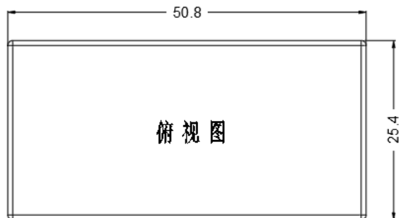
标准型 50.8*25.4*12.7mm
