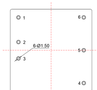
推荐PCB开槽尺寸
