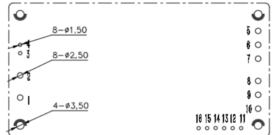
推荐PCB开槽尺寸
