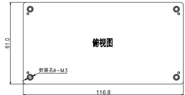
标准型 116.8*61*12.7mm
