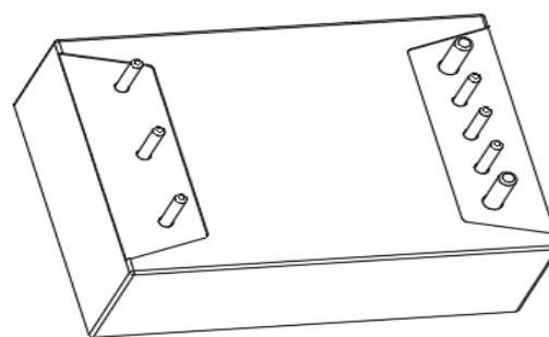
散热铝盖型 34.3*24.1*11.7mm
