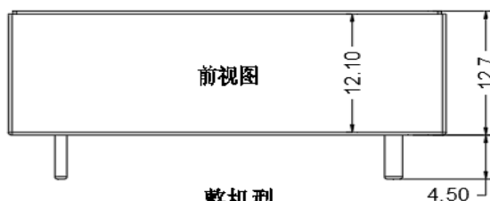
整机型 36.7*26.5*12.7mm
